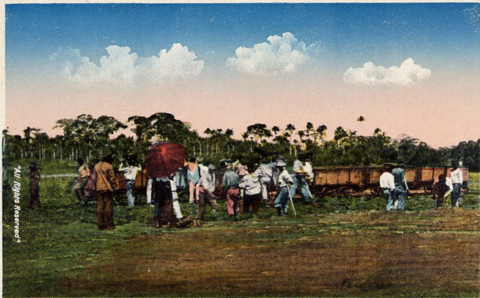
Pitch Lake, Trinidad. B. W. I.
